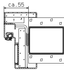
bekleidetes Stahlprofil
